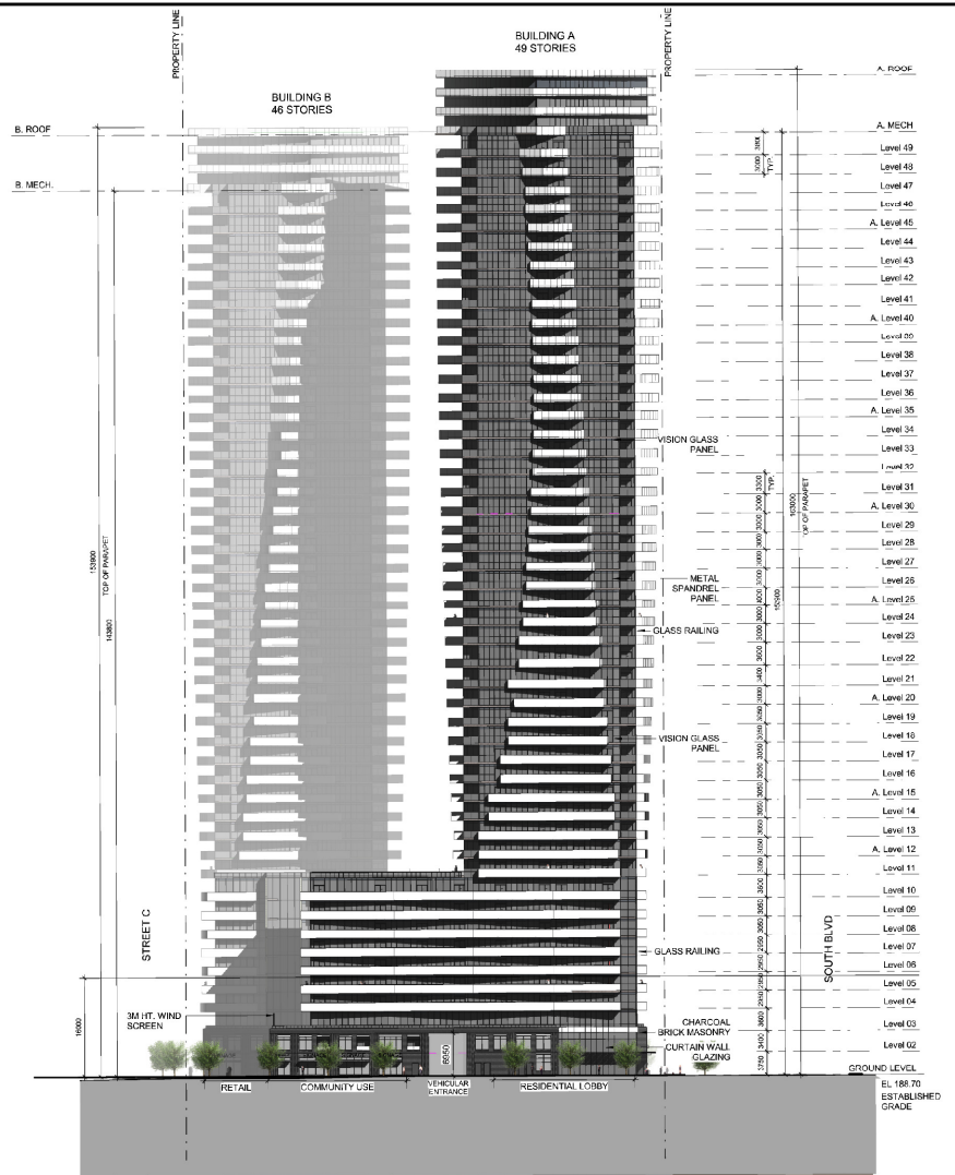
1 WEST ELEVATION A402 Scale: 1 : 400
